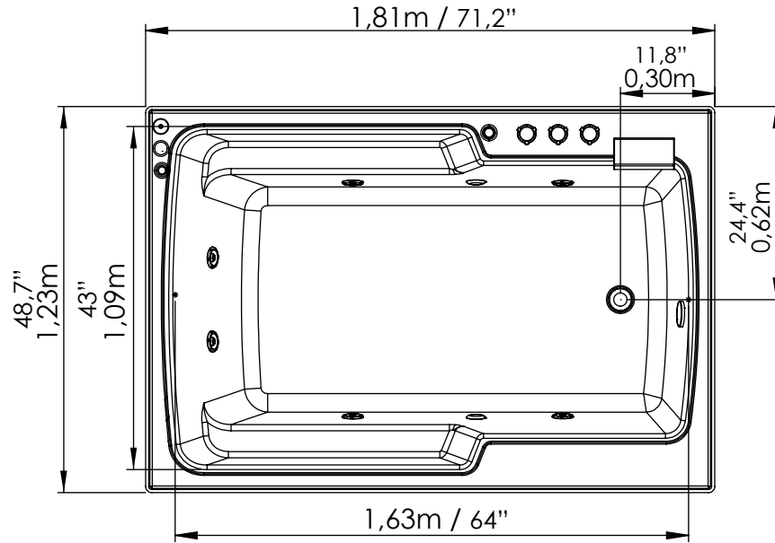
VISTA EN PLANTA / PLANT VIEW
