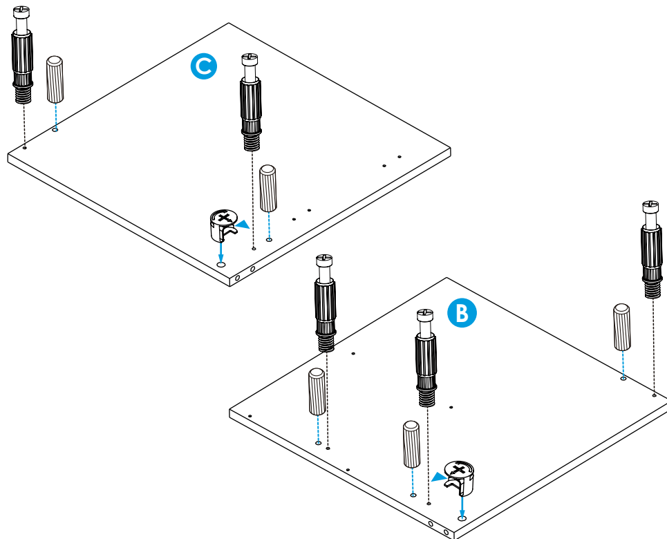
Minifix Minifix cams
